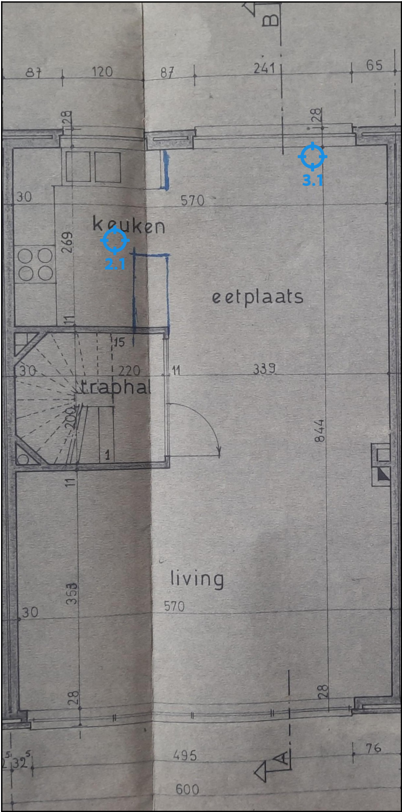
Legende van plan 1.3: Plan 1ste Verdieping
